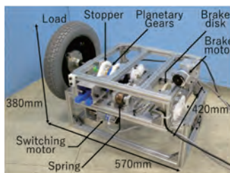
図2 実験装置外観
