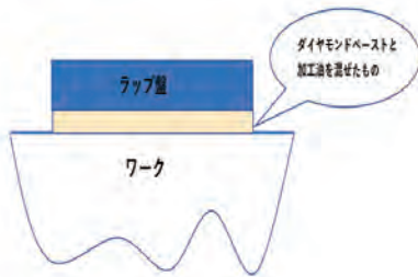
図 1. ハンドラップの仕組み
