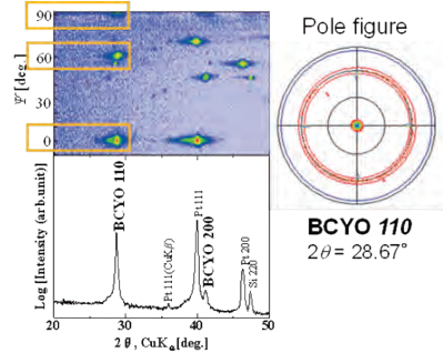
図 高度に110配向したBCYO電解質薄膜のX線回折結果
