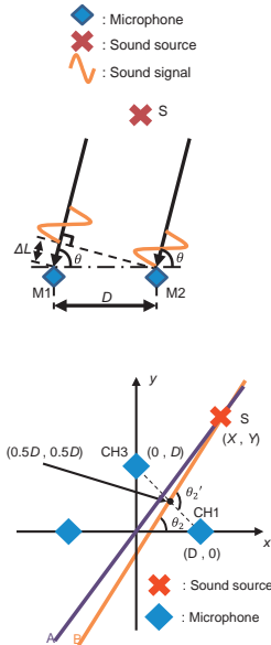
音源位置推定のための提案法
