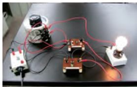
小型化した実習装置
