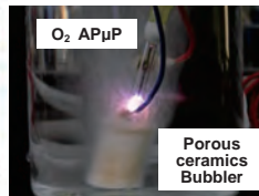
図4 プラズマ・バブリング水処理
