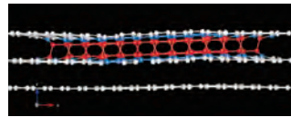
図1: グラファイト中に光誘起されたダイヤモンドドライクドメイン (Diaphite)の構造(数値計算結果)
