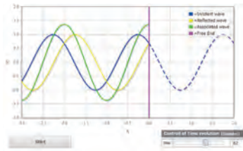
図4: 正弦波の自由端反射
