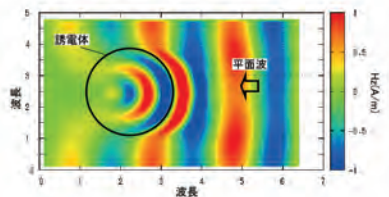
図3 FDTD 法による計算例
