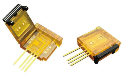
パッケージ変換ソケット (TOシリーズ)
