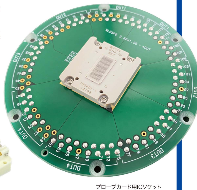
プローブカード用ICソケット
