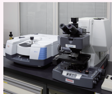
フーリエ変換赤外分光光度計★
